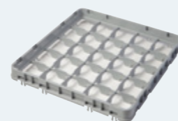
AUFSATZ MIT 25 FÄCHERN 25E2 max Ø 8,7 cm / Passend für Basiskorb (blau) 25S318168 / 50 x 50 x 4,2 cm
